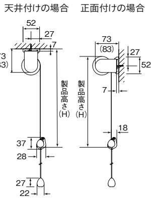
標準プルコードタイプ (マイテック)
