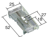
標準プルコードタイプ/標準チェーンタイプ/標準ワンタッチチェーンタイプ
