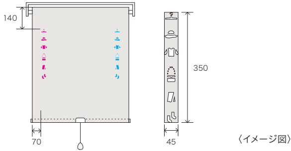
標準プルコードタイプ TR-6033 / マテリアルグレー / オプション: ポイントカット TYPE305
