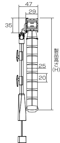
コルトブラインド25Ⅱ 浴窓テンションワンポールタイプ
