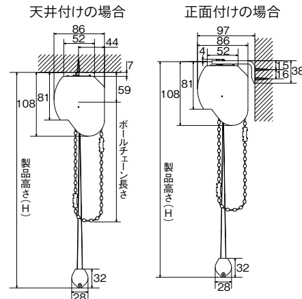
ビジックデコラ(フロントカバー付きチェーンタイプ)
