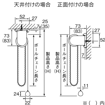
標準チェーンタイプ/ワンタッチチェーンタイプ (マイテックループ/マイテックワンタッチループ)
