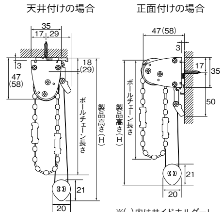
ビジック小窓(チェーンタイプ)
