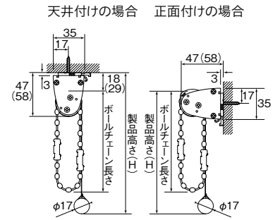
小窓チェーンタイプ (マイテックループ小窓)
