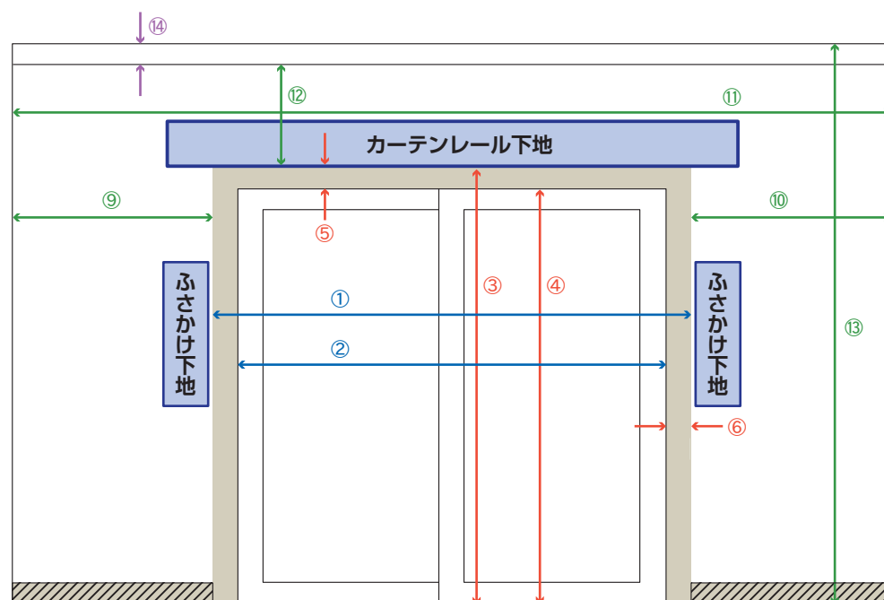
(正面)
