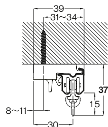
天井付シングルブラケット付 (ブラケット幅=32mm)
