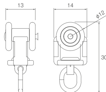
ランナー寸法図（単位：mm）
