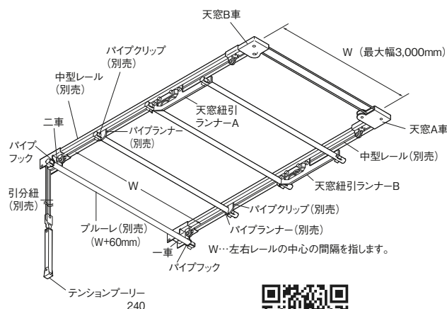
天窓紐引部品セット組立図
