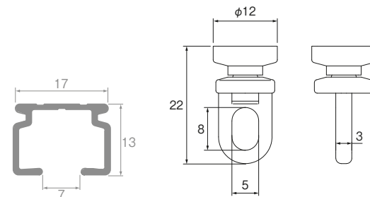
レール断面図 (単位: mm)
