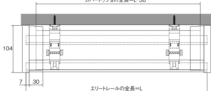
カバートップⅡセット平面図
