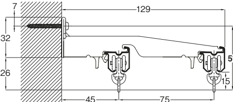
エキストラダブルブラケット付 (ブラケット幅=18mm)
