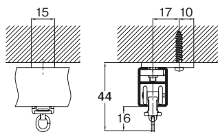
壁面ブラケットA付
