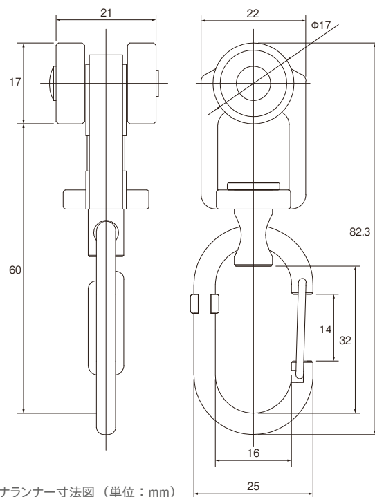
カラビナランナー寸法図（単位：mm）
