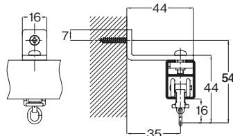
壁面ブラケットB付
