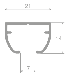
レール断面図 (単位: mm)
