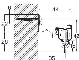
シングルブラケット付 (ブラケット幅=18mm)
