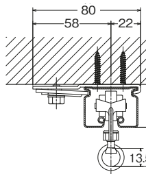
天井シングルブラケット付 (特殊ランナー)
