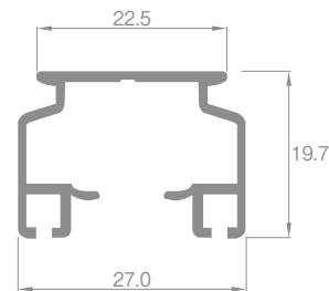
レール断面図（単位：mm）
