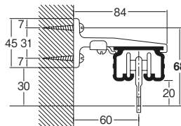
シングルブラケット付 （ブラケット幅＝34mm） （ランナー使用）
