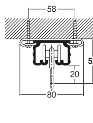
天井付シングルブラケット付 （ブラケット幅＝38mm） （ランナー使用）
