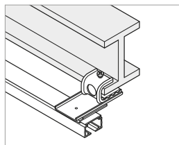
H鋼から持ち出して取付
