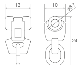
ランナー寸法図 (単位: mm)
