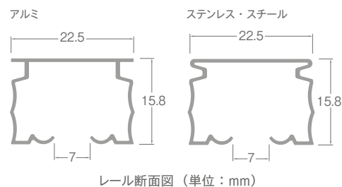
レール断面図 (単位: mm)
