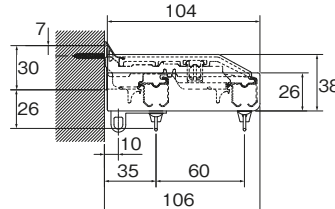
カバートップⅡセット側面図
