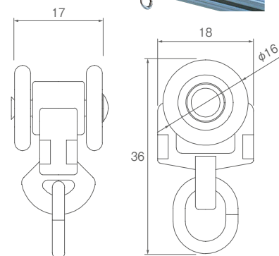
ランナー寸法図 (単位: mm)
