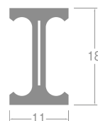
レール断面図 (単位: mm)
