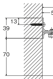
シングルブラケット付 (カラビナランナー)
