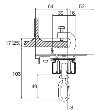
天井付シングルブラケットM 2 付（H鋼の下） （カラビナランナー使用）
