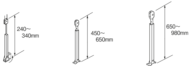
テンションプーリー 240
