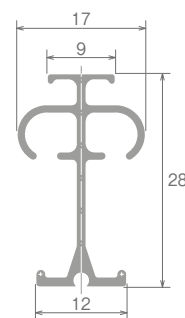
レール断面図（単位：mm）
