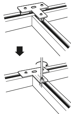
T型止め金具
