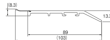
カバートップⅡ本体側面図
