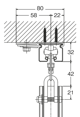
天井シングルブラケット付 (特殊ランナー+ 間仕切サイドポール+U継金具) (間仕切中間ポール+U継金具)
