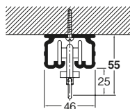
天井直付 （スイングランナー使用）
