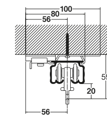
天井付シングルブラケットM 2 付 （ブラケット幅＝55mm） （ランナー使用）
