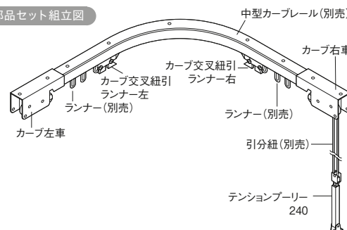
カーブ紐引部品セット組立図
