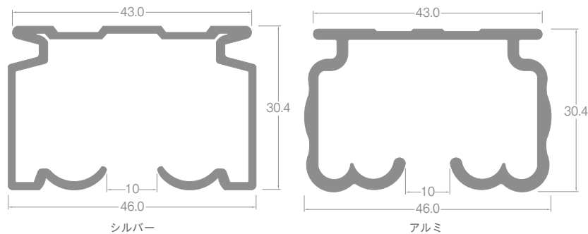
レール断面図 (単位: mm)
