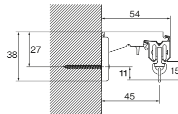
LTダブルブラケット付 (ブラケット幅=35mm)
