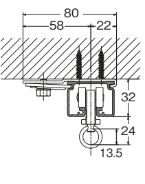
天井シングルブラケット付 (ランナー)
