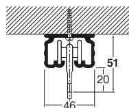
天井直付 （ランナー使用）
