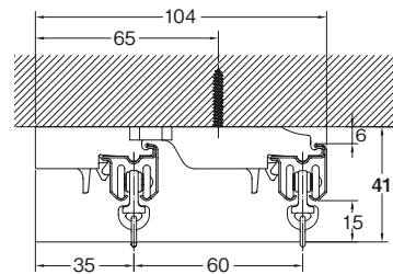
天井付ダブルブラケットⅡ付 (ブラケット幅=21mm)
