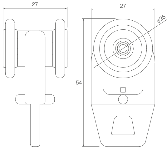
ランナー寸法図 (単位: mm)
