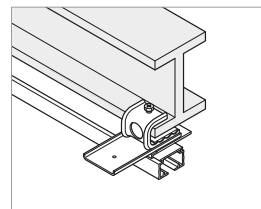
H鋼の下に取付
