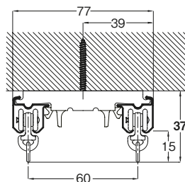
天井付ダブルブラケット付 (ブラケット幅=18mm)
