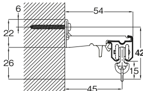
エキストラシングルブラケット付 (ブラケット幅=18mm)
