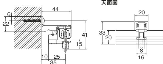
カバートップⅡセット平面図
