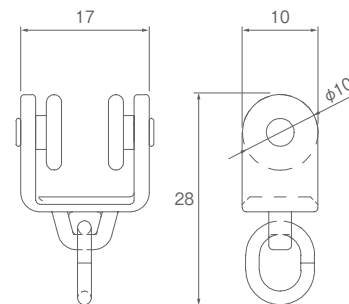
ランナー寸法図 (単位: mm)
