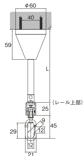
固定吊棒セット (カラビナランナー使用時)
