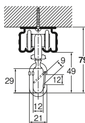
天井付シングルブラケットM 2 付（持ち出し） （カラビナランナー使用）
