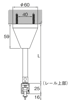
固定吊棒セット
