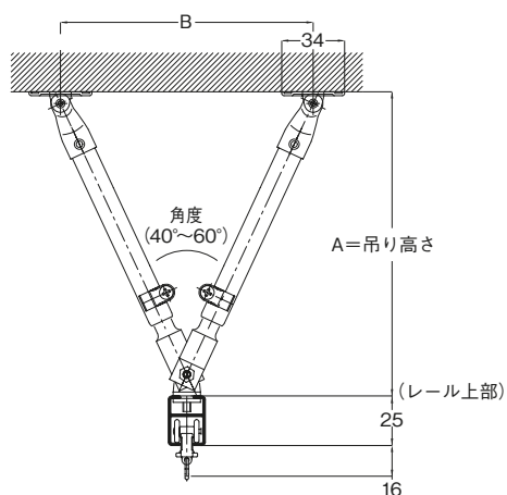
伸縮吊棒A (カラビナランナー使用時)
