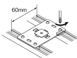
ダブル止め金具C
