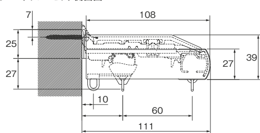
カバートップⅡセット側面図
