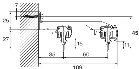
ダブルブラケット付（ブラケット幅=18mm）
