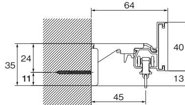
LTダブルブラケット付（ブラケット幅＝35mm）
