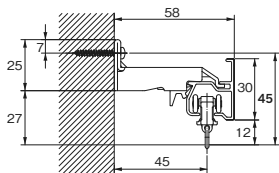
エキストラシングルブラケット付 （ブラケット幅=18mm）
