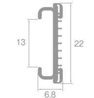
レール断面図(単位:mm)
