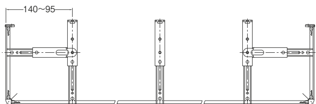
基本取付図
