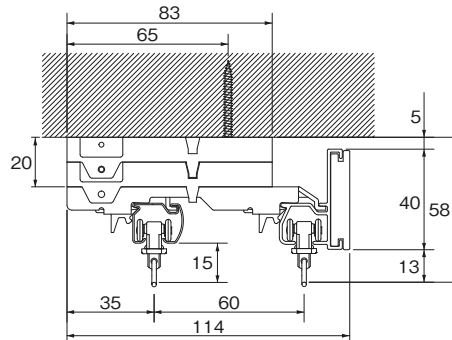
カバートップⅡ MC セット側面図
