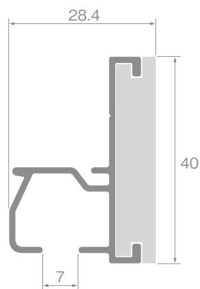
レール断面図 (単位：mm)
