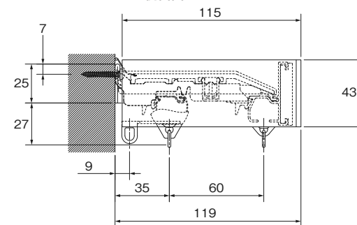
カバートップⅡ MC セット側面図
