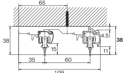
天井付ダブルブラケット付（ブラケット幅=19mm）
