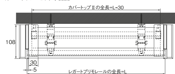
カバートップⅡセット平面図
