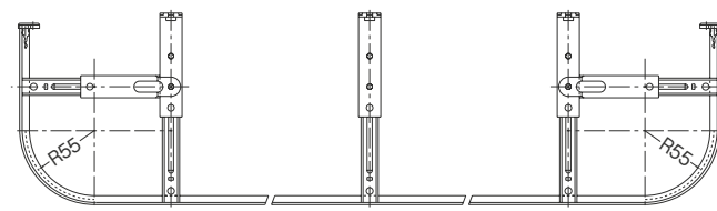
基本取付図
