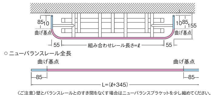
基本取付図
