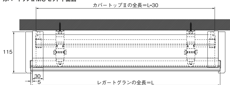
カバートップⅡ MC セット平面図
