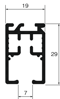
レール断面図（単位：mm）
