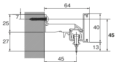
ダブルブラケット付（ブラケット幅＝18mm）
