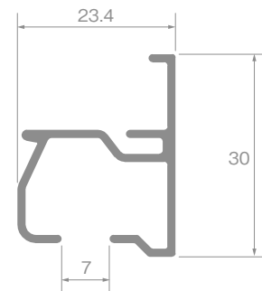
レール断面図 (単位: mm)
