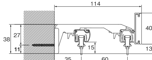
LTダブルブラケット付（ブラケット幅＝35mm）
