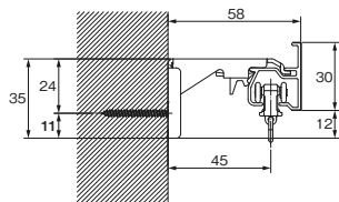
LTエキストラシングルブラケット付 （ブラケット幅=35mm）
