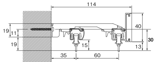
NTダブルブラケット付（ブラケット幅＝44mm）
