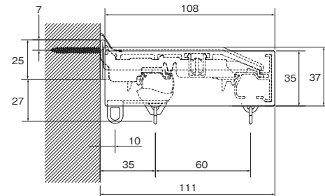
本体側面図
