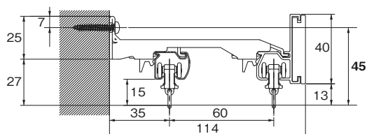
NTダブルブラケット付（ブラケット幅＝44mm）
