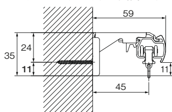
LTエキストラシングルブラケット仕様（ブラケット幅=35mm）
