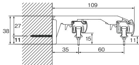
LTダブルブラケット付（ブラケット幅=35mm）
