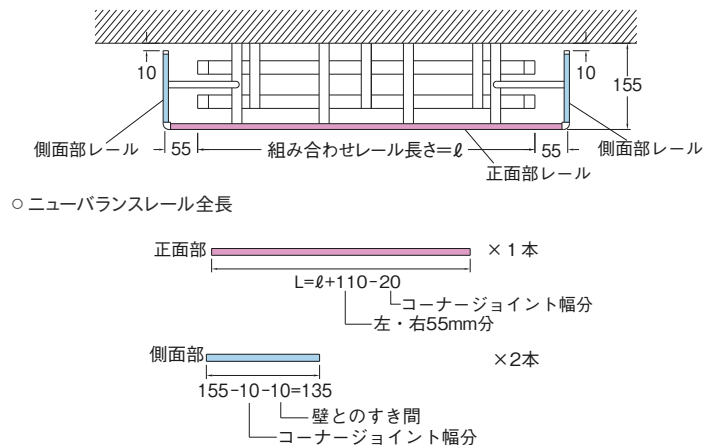
基本取付図
