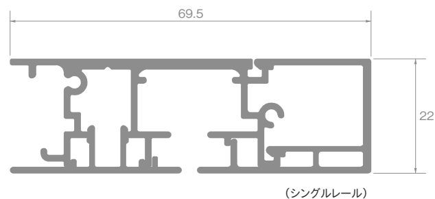
レール断面図 (単位: mm)
