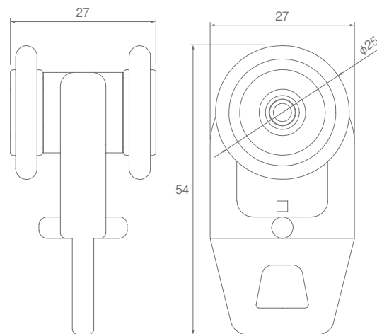
ランナー寸法図 (単位: mm)
