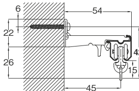
エキストラシングルブラケット付（ブラケット幅=18mm）
