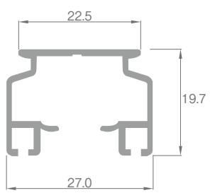
レール断面図 (単位: mm)
