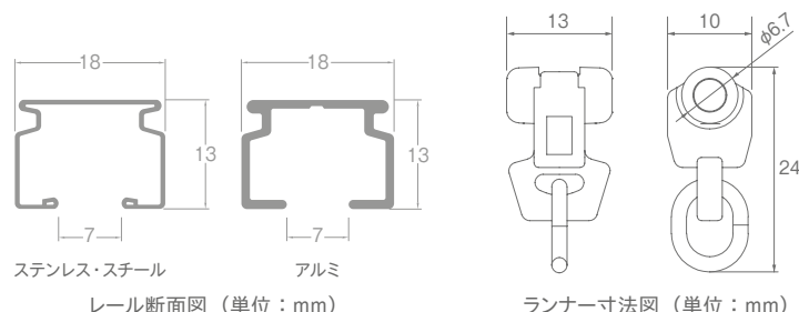
レール断面図 (単位: mm)
