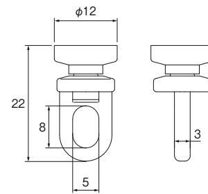
ランナー寸法図 (単位: mm)
