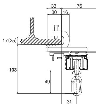
天井付シングルブラケットM 2 付（持ち出し） （カラビナランナー使用）
