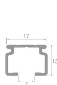
レール断面図 (単位: mm)
