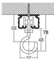
クリップ付ブラケットプレート使用 ※（ ）はクリップ付ブラケットプレートMの場合
