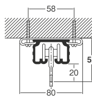
天井付シングルブラケット付 （ブラケット幅＝38mm） （ランナー使用）
