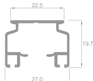
レール断面図（単位：mm）
