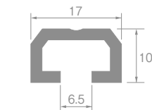
レール断面図 (単位: mm)
