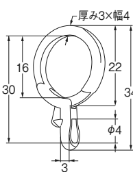
寸法図 (単位: mm)
