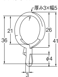
寸法図 (単位: mm)
