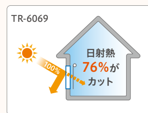
ロールスクリーンを付けた場合 複層ガラス窓 + ロールスクリーン \eta = 0.24 (TR-6069)
