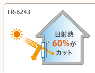
ロールスクリーンを付けた場合 複層ガラス窓 + ロールスクリーン \eta = 0.4 (TR-6243)
