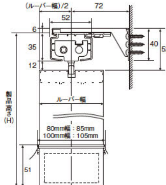
正面付け (正面付ブラケット使用)
