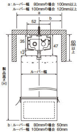
カーテンボックスの内側に取付ける場合
