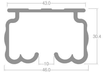
レール断面図（単位：mm）
