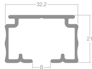
レール断面図（単位：mm）
