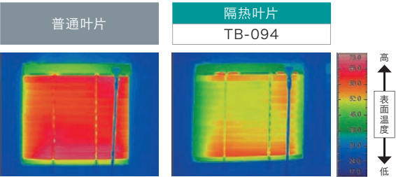
百叶窗整体吸收热量，并进行散热。 ※向百叶窗背面照射4只150W反射节能灯泡时的热成像对比（从百叶窗正面拍摄）
