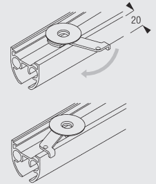
3825 クランプ
